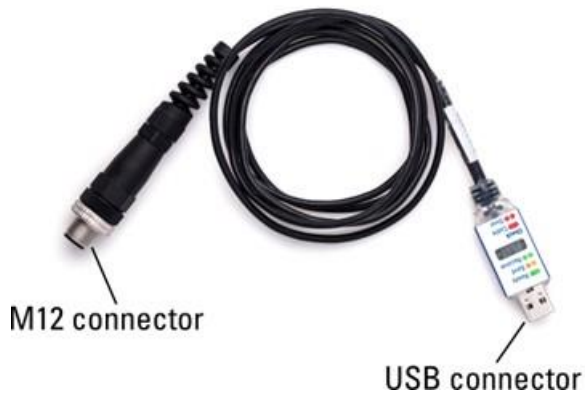
Figuur 2 De connectoren van de Smart Interface Cable.
