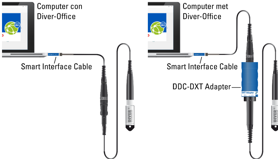
Figura 3 Smart Interface Cable conectado a (izquierda) un DXT-cable y (derecha) a un cable de datos Diver a través del adaptador DDC-DXT Adapter (AS348).
