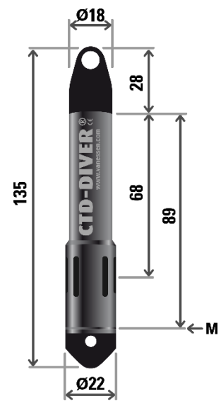
M = membrana Dimensiones in mm
