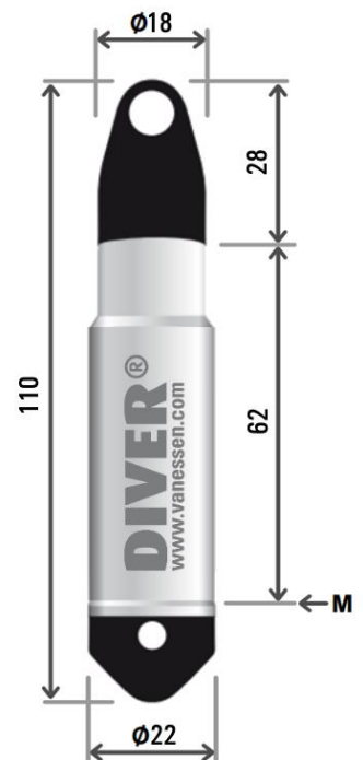
M = membrana Dimensiones en mm
