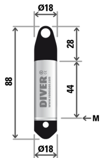
M = membrana Dimensiones in mm
